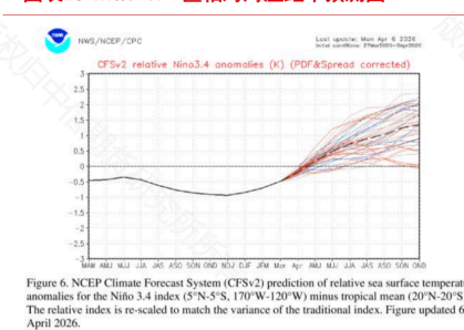
图表2: Niño 3.4 区相对海温距平预测图
